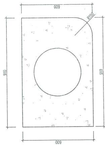
MẶT BẰNG
