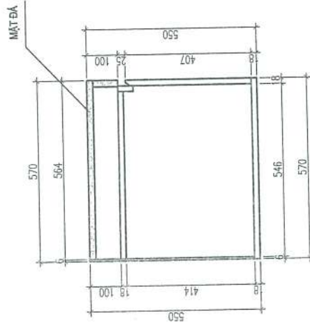
MẶT CẮT 1-1
