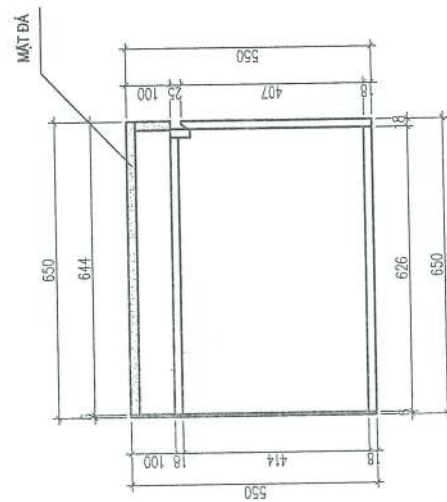
MẶT CẮT 1-1
