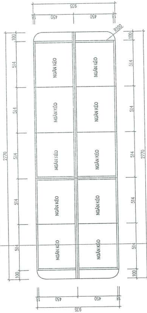
MẶT BẰNG
