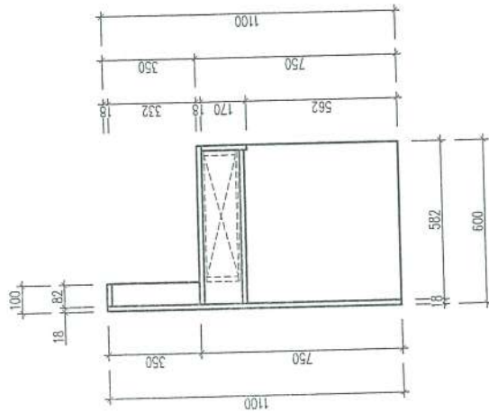
MẶT CẮT 1-1
